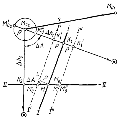
Рис. 115. Получение обсервованного места при разновременных наблюдениях Солнца
