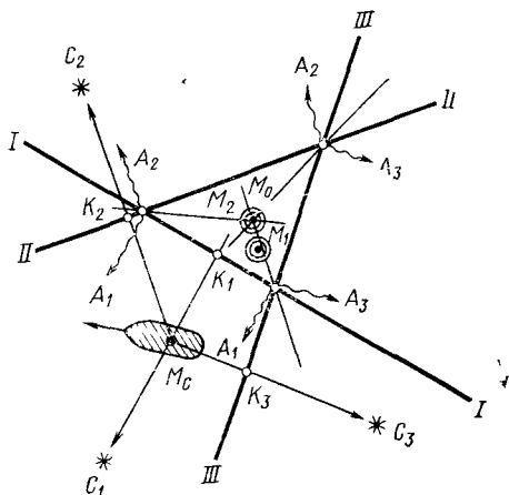
Рис. 109. Нахождение обсервованного места при учете систематических ошибок в высотах, когда светила расположены по всему горизонту
