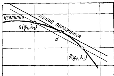
Рис 84 Изображение изолиний и линий положения
