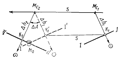
Рис. 115. Получение обсервованного места при разновременных наблюдениях Солнца
