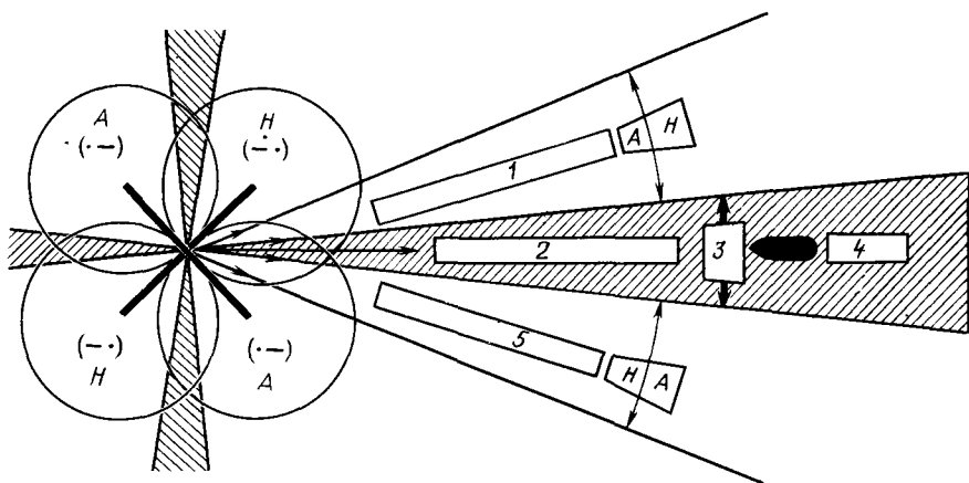
Рис 108 Створный радиомаяк
