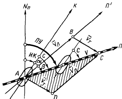
Рис. 64 Учет совместного сноса ветром и течением
