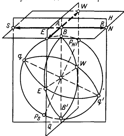
Рис. 4. Основные линии и плоскости на земном шаре
