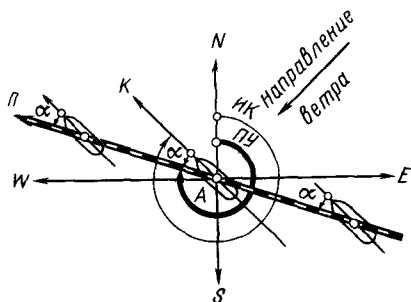
Рис 62 Учет сноса ветром
