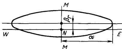
Рис. 18. Незатухающие колебания главной оси гироскопа
