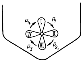
Рис 156 Сила струи «на бросывания»
