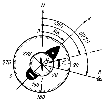
Рис 102 Картушка радиопеленгатора
