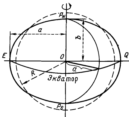
Рис. 2. Основные точки и круги на земном шаре
