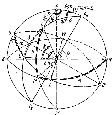
Рис. 83. Небесная сфера
