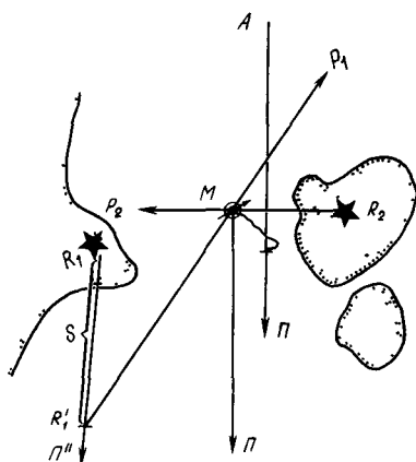
Рис 103 Радиопеленгование на «малых» расстояниях
