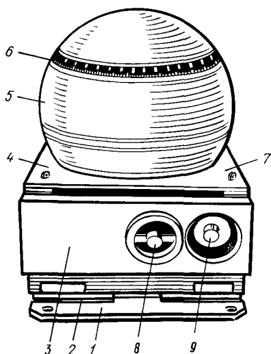
Рис. 20. Внешний вид гироазимуткомпаса «Вега»:
