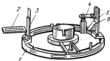
Рис. 24. Пеленгатор: 1 — основание; 2 — откидное зеркало; 3 — предметная мишень; 4 — набор свето-фильтров; 5 — глазная мишень, призма
