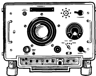
Рис. 99. Радиопеленгатор «Румб»
