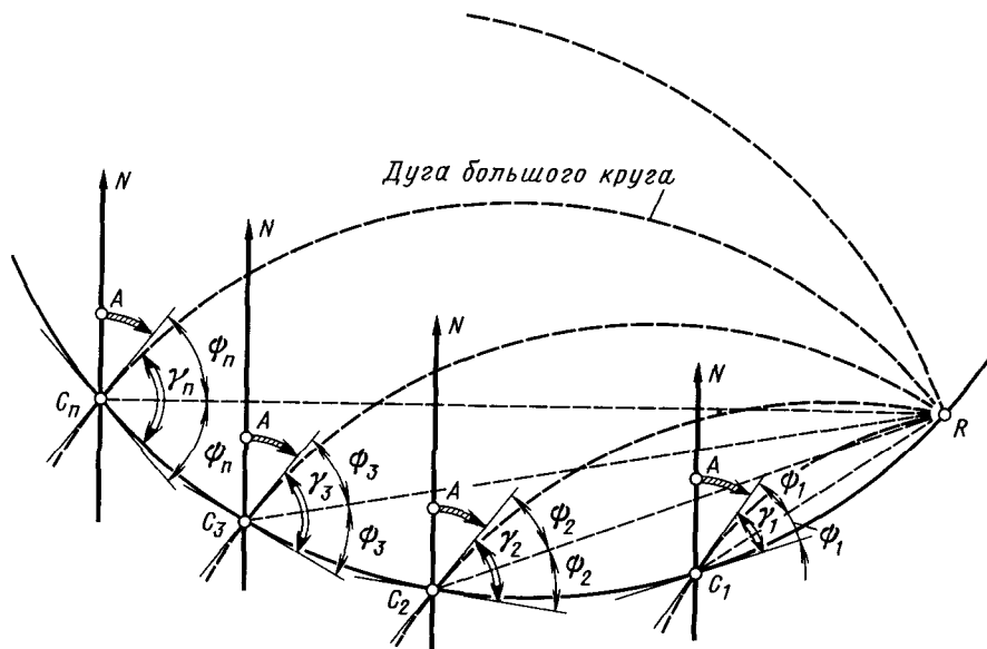
Рис. 74. Три замечательные линии на меркаторской проекции положения
