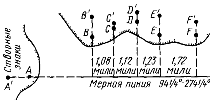
Рис 9 Мерная линия
