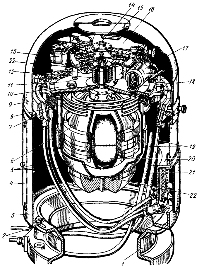
Рис. 19. Основной прибор гироскопа «Курс»:
