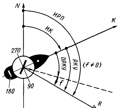
Рис 101 Истинный радиопеленг (ИРП) при f \neq 0
