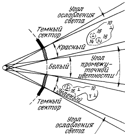
Рис. 37. Секторный огонь
