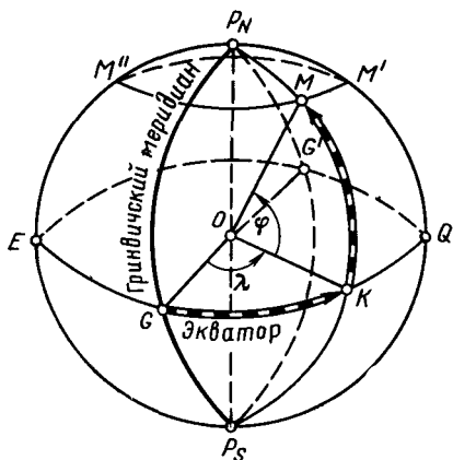
Рис. 1. Форма и размеры Земли
