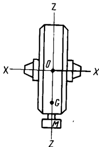
Рис. 16. Превращение гироскопа в гироскопический компас
