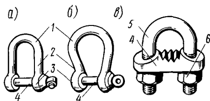
Рис. 128. Скобы:
