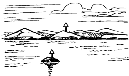
Рис. 36. Вождение по створу: курс должен быть изменен влево
