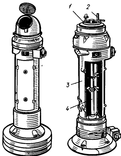
Рис. 25. Магнитный компас: 1 — котелок; 2 — пеленгатор; 3 — нактоуз, 4 — девиационный прибор
