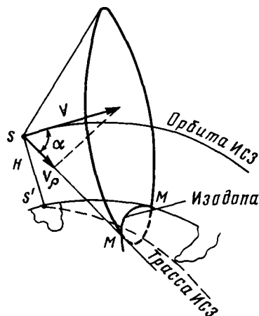
Рис 110. Эффект Доплера
