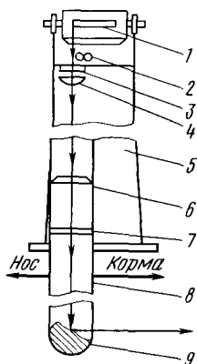
Рис 26 Магнитный компас КМО-Т 1 — картушка, 2 — осветительная лампа 3 — защитное стекло, 4 — верхняя линза 5 — нактоуз, 6 — нижняя линза, 7 — обогривательное стекло 8 — труба оптической системы, 9 — зеркало
