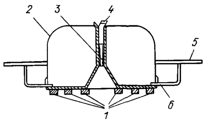
Рис. 23. Картушка с поплавком: 1 — система магнитных стрелок; 2 — поплавок; 3 — топка; 4 — винт для крепления; 5 — диск; 6 — кронштейны
