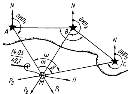
Рис 76 Метод пеленгов трех ориентиров
